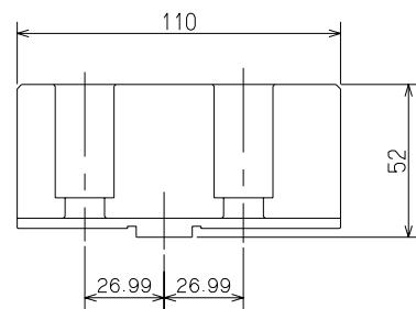
ソフトジョー SOFT JAW
